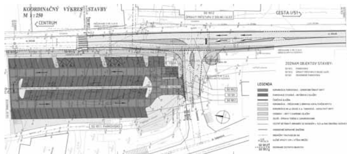
Koordináčný výkres stavby FOTO ARCHÍV MŠÚ
