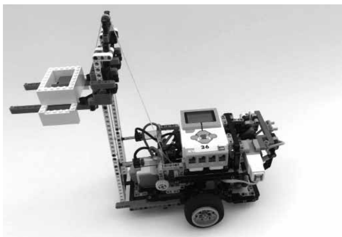
Dialkovo ovládaný vysokozdvíhny vozík FOTO ARCHÍV AUTORA
