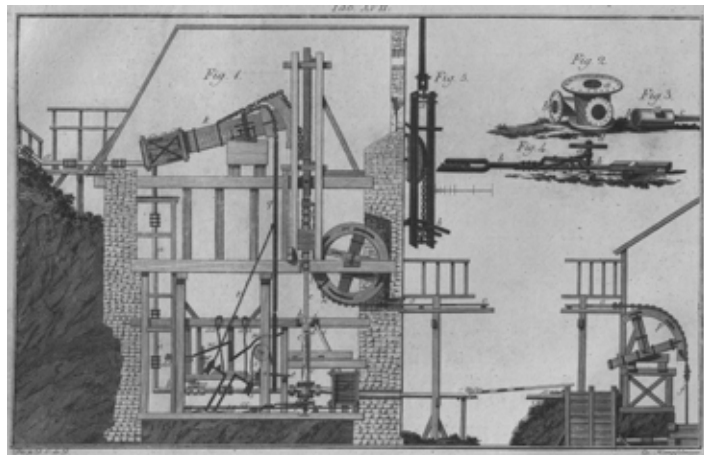
Vodnostlpcový čerpací stroj J. K. Hella, namontovaný v roku 1759
