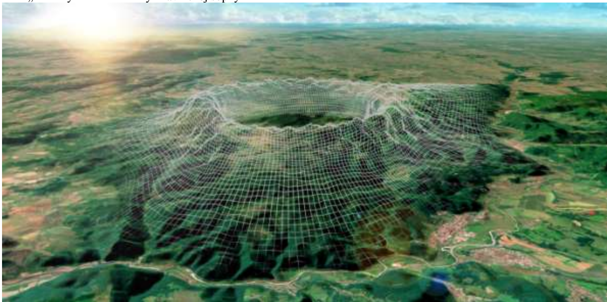
Obr: „Drôtený“ model kaldery štiavnickej sopky
