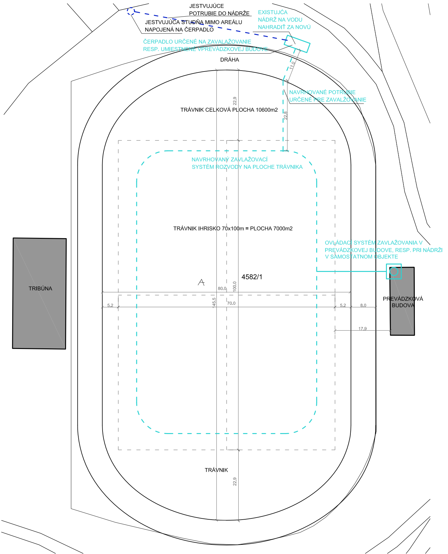
SITUÁCIA M 1 : 750
